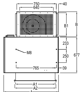
Вид снизу Без клапана воздушного
