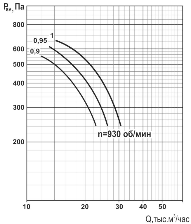
ВКР2ДУ-9
