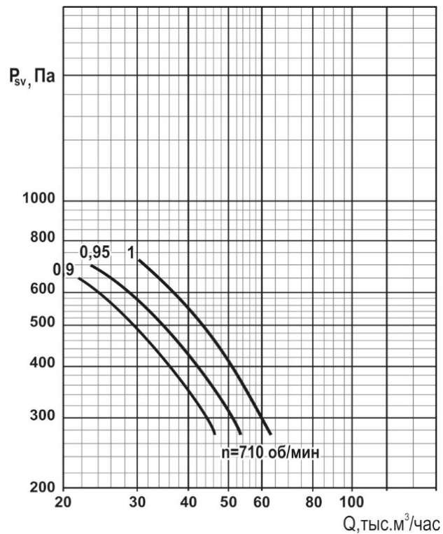
ВКР2ДУ-12,5
