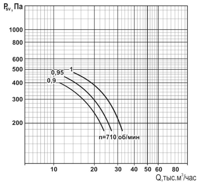
ВКР2ДУ-10
