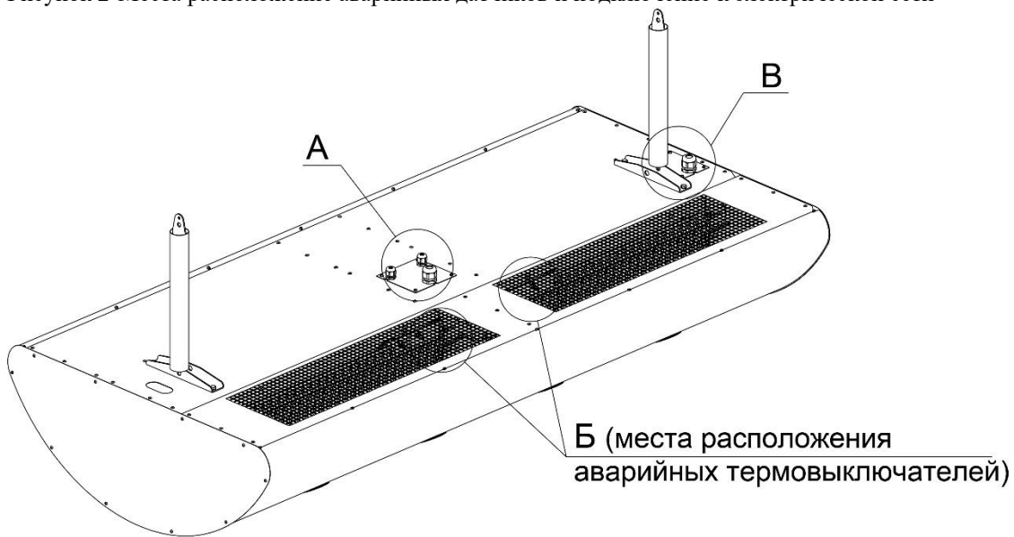
Рисунок 2-Места расположение аварийных датчиков и подключение к электрической сети
