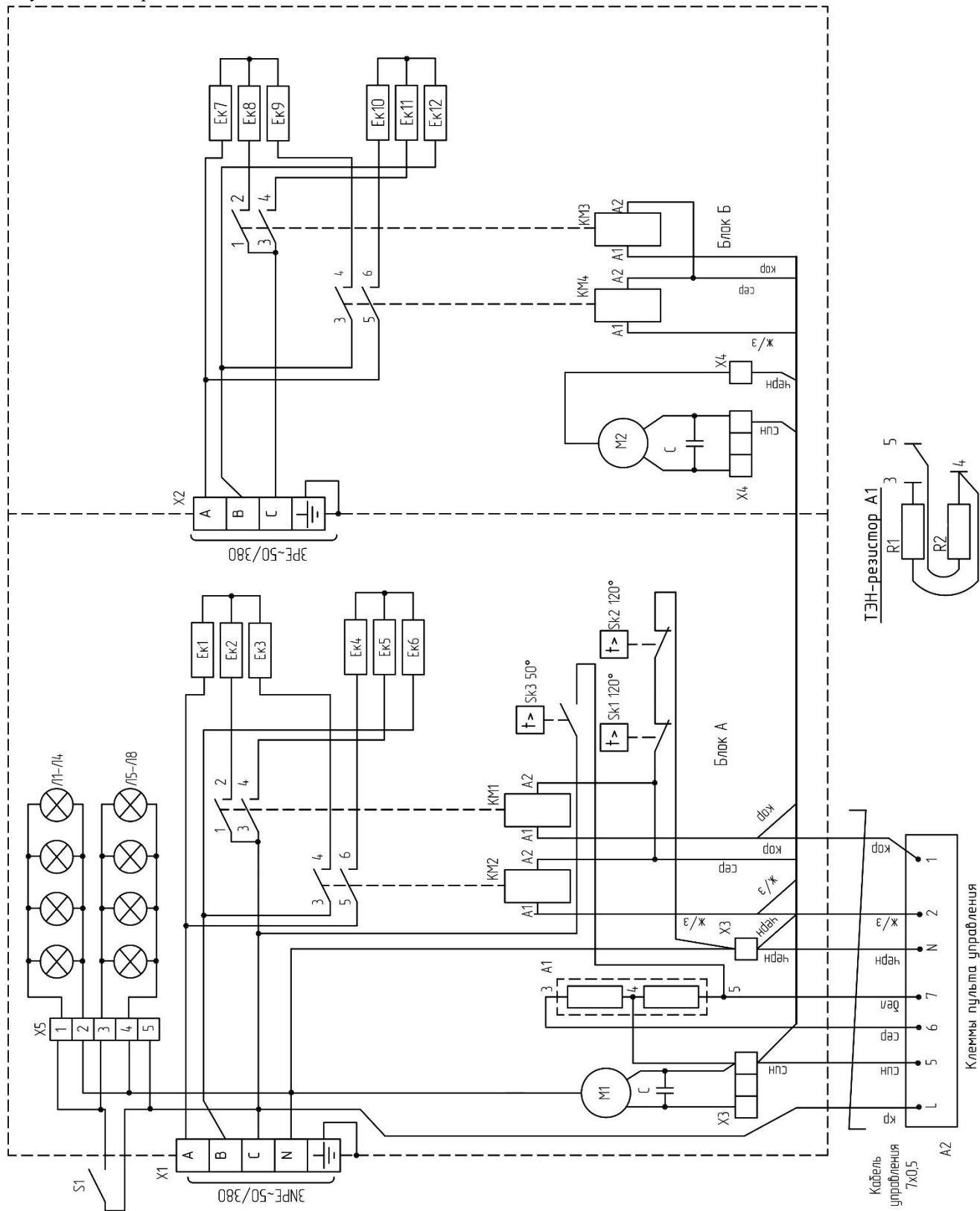
Рисунок 5-Электрическая схема КЭВ-24П6053Е, КЭВ-36П6053Е
