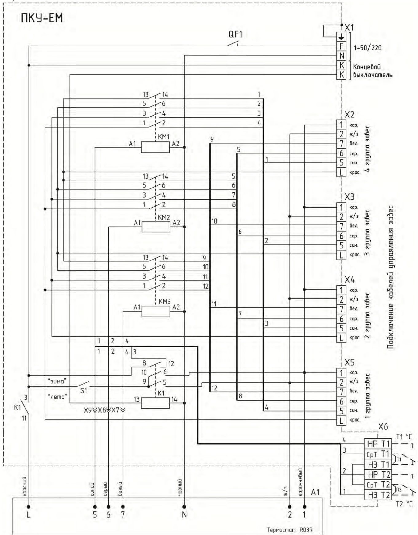
Рисунок 9-Электрическая схема пульта коммутации и управления для завес с электрическим источником тепла (ПКУ-ЕМ).
