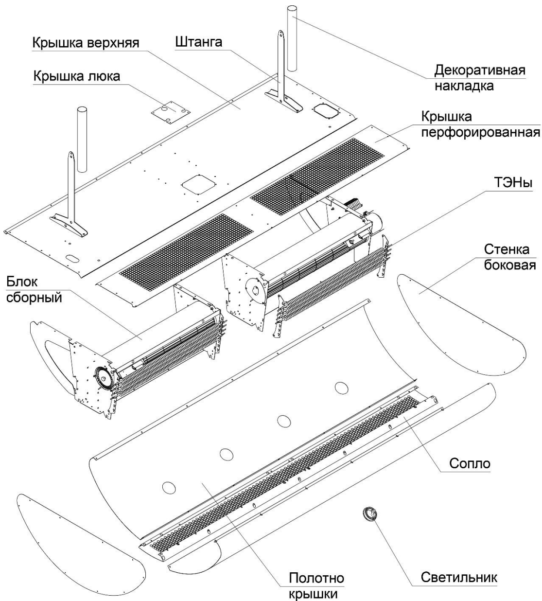
Рисунок 1-Интерьерная воздушно-тепловая завеса «Линза»
