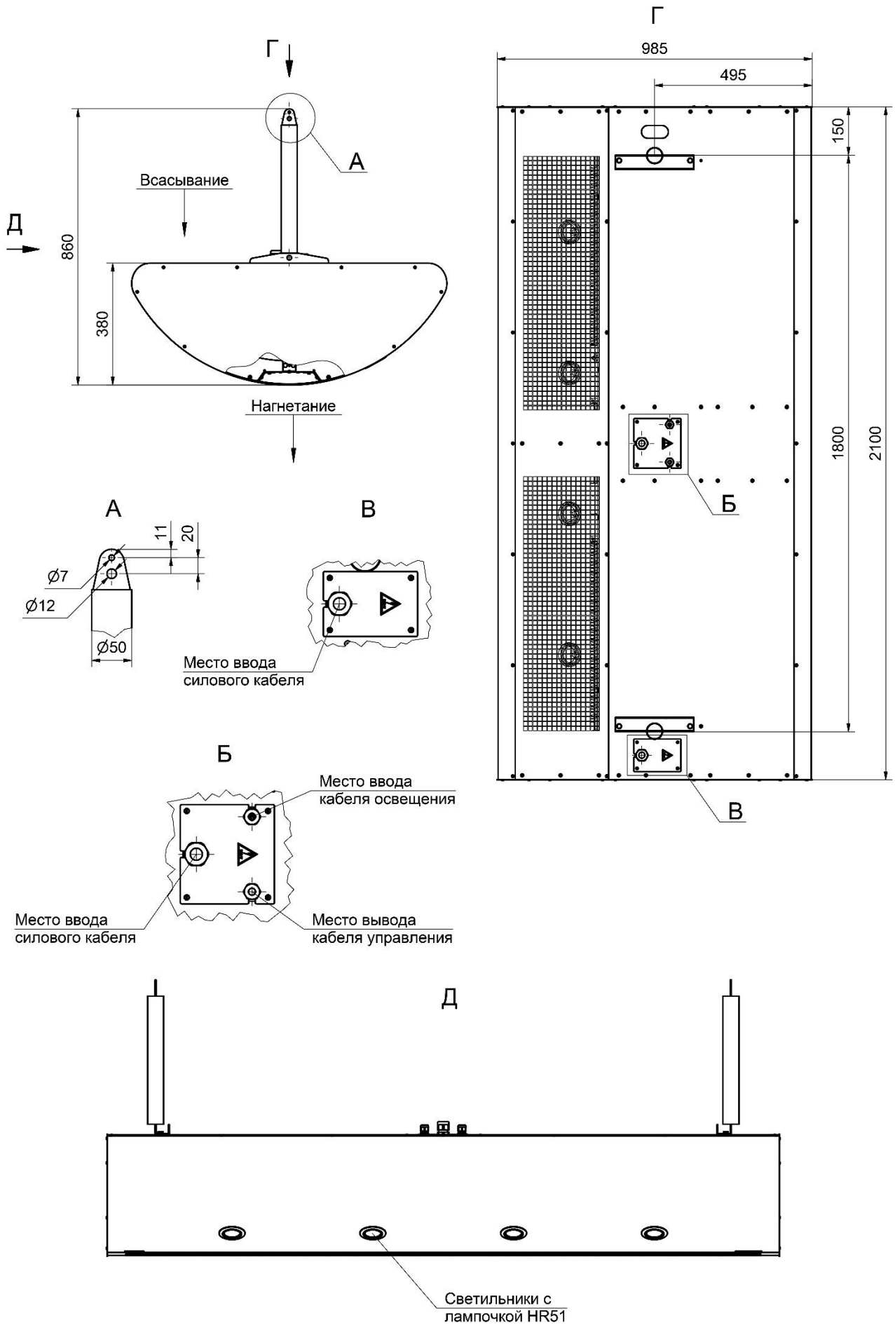
Рисунок 4-Габаритные и крепежные размеры
